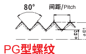
德制PG螺纹 DIN 40430
