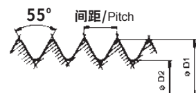
英制G管螺纹 DIN ISO 228
