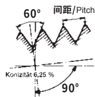
美制NPT锥螺纹
